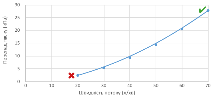
Падіння тиску гарячої води (з боку корпусу)
